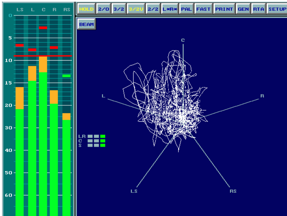
Bild 2.2 Multikanal Audiometer (LAY Audio) Beschreibung siehe HOEG/GRUNWALD [49]
